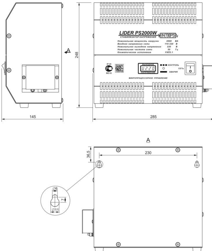
Габаритные и установочные размеры стабилизаторов напряжения переменного тока LIDER PS2000W-50
