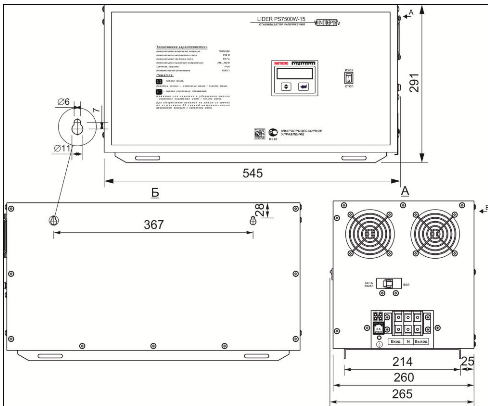
Габаритные и установочные размеры стабилизаторов напряжения переменного тока LIDER PS10000W-15
